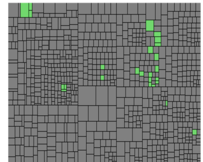
FlatMapTest.testFlatMap
